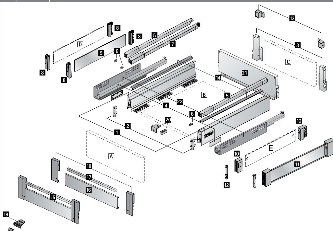
Сборочный чертёж
